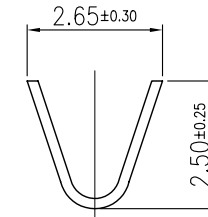
A-A SECTION
